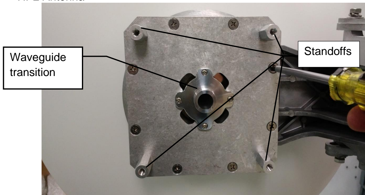
HP2 Antenna
